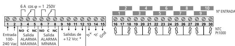
Ejemplo de conexionado de otras sondas:
